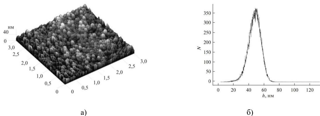
Рисунок 1 – а) 3D АСМ – изображение наноструктур \text{Ga}_x\text{In}_{1-x}\text{As} -GaAs полученных методом ИЛО; б) зависимость количества островков (N) от их размера (h) [а) 3D AFM image of \text{Ga}_x\text{In}_{1-x}\text{As} -GaAs nanostructures obtained by the ILO method; b) dependence of the number of islands (N) on their size (h)]
