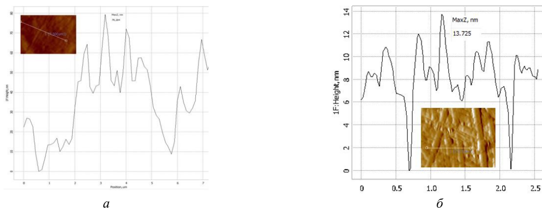
Рисунок 2. Профиль сечения с фрагментом АСМ-изображения: а – образца 1; б – образца 2 Figure 2. Section profile with fragment of AFM-image: a – sample 1; b – sample 2
