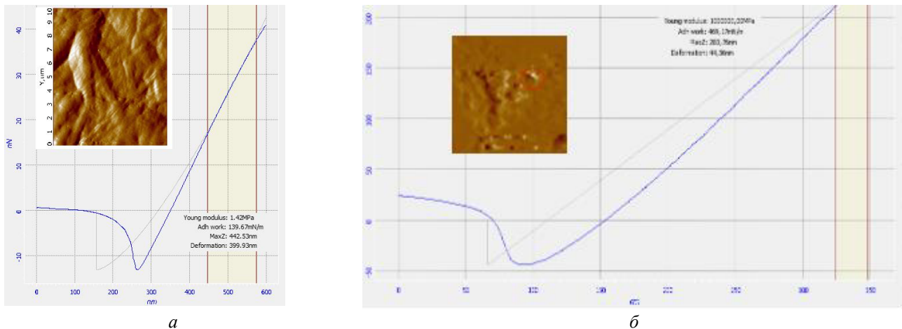
Рисунок 4. Силовые кривые образца 3 с фрагментом области исследования: а – модуль Юнга = 1,43 МПа, деформация = 399,93 нм; б – модуль Юнга = 1000000 МПа, деформация = 44,36 нм Figure 4. Force curves of the sample 3 with a region fragment: a – Young's module = 1,43 МПа, deformation = 399,93 нм; б – Young's module = 1000000 МПа, deformation = 44,36 нм
