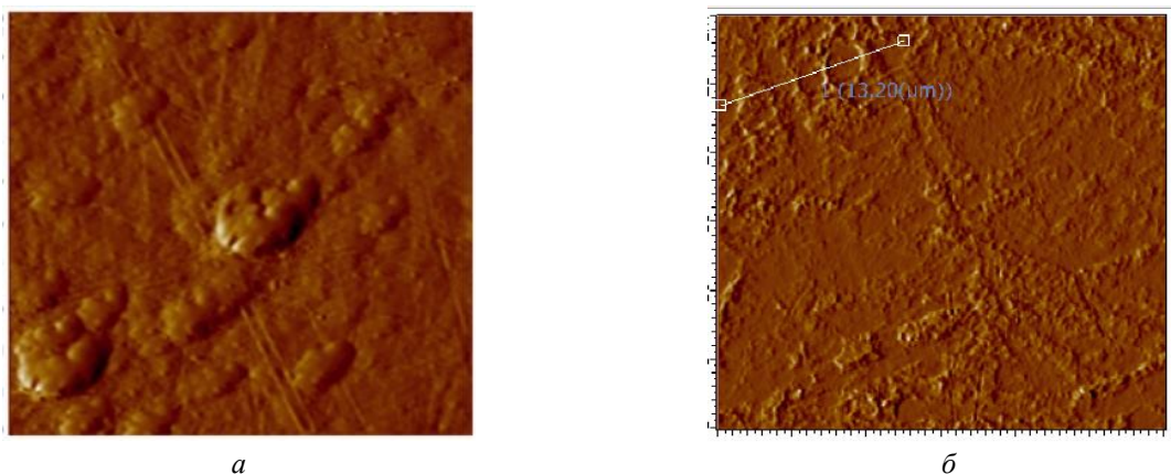
Рисунок 3. Фрагмент АСМ-изображения размером 10x10, образец 3: а 3 – топография; б – фаза Figure 3. Fragment of AFM-image scale 10x10 nm, sample 3: a 3 – topography; b – phase
