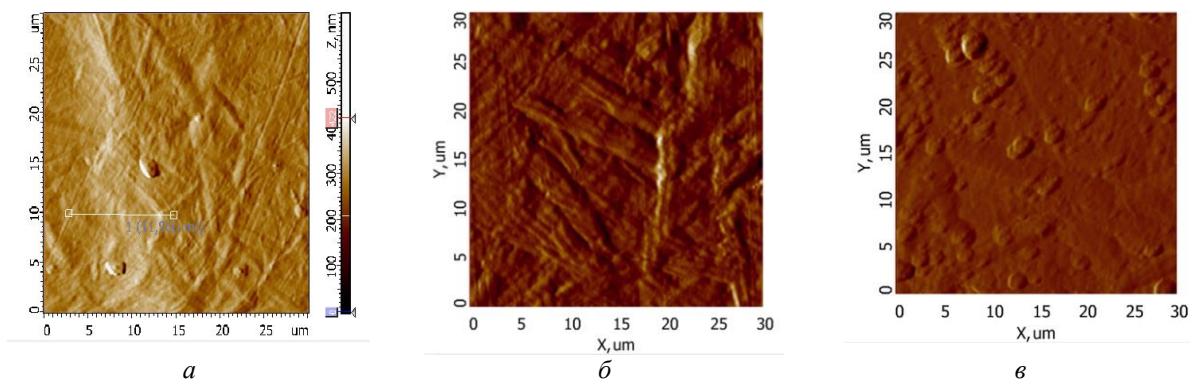
Рисунок 1. АСМ-изображения поверхности образцов, размер скана 30x30 мкм: а – образец 1; б – образец 2 1 ; в – образец 3
