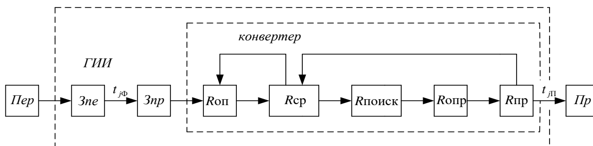
Рисунок 1 – Блок-схема ГИИ ( З_{пр} – блок запроса приемника; З_{пе} – блок запроса передатчика; Пр – блок приема; ( R_{опр} ) – блок определения систем кодирования источника и приемника; ( R_{ср} ) – блок сравнения; ( R_{поиск} ) – блок поиска; ( R_{оп} ) – блок оптимизации; ( R_{пр} ) – блок преобразования; ( R_{пров} ) – блок проверки; Пер – блок передачи) [Flowchart flexible intelligent interface ( З_{пр} – receiver request block; З_{пе} – transmitter request unit; Пр – receiving unit; ( R_{опр} ) – source and receiver coding system detection unit; ( R_{ср} ) – comparison block; ( R_{поиск} ) – search block; ( R_{оп} ) – optimization block; ( R_{пр} ) – conversion unit; ( R_{пров} ) – check block; Пер – transmission unit)]
