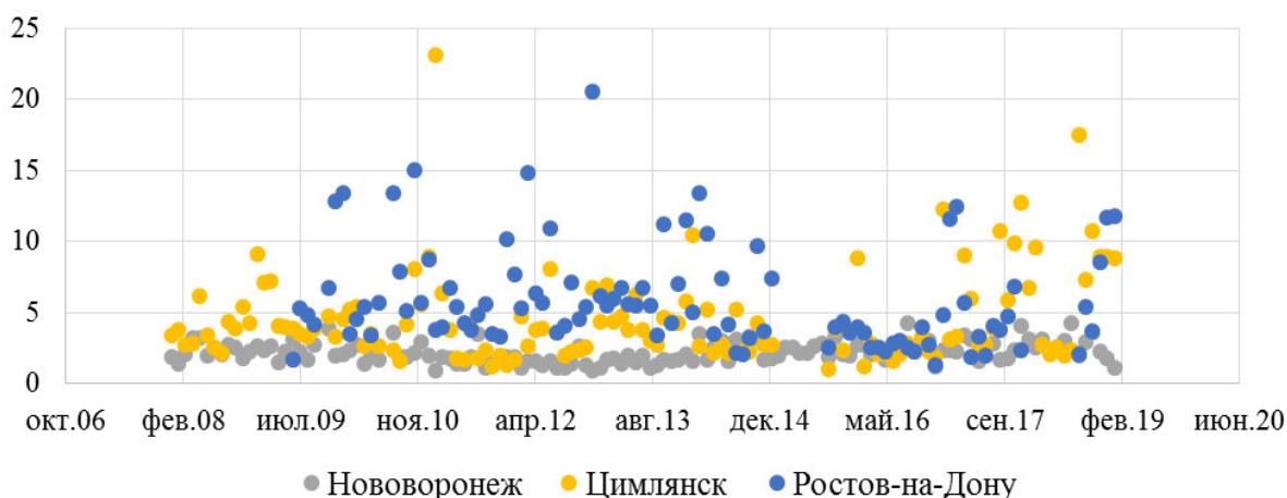
Рисунок 2 – Максимальные ежемесячные значения суммарной \beta -активности атмосферных выпадений, Бк/(м 2 ·сутки) [The maximum monthly values of the total \beta -activity of atmospheric precipitation, Bq / (m 2 · day)]
