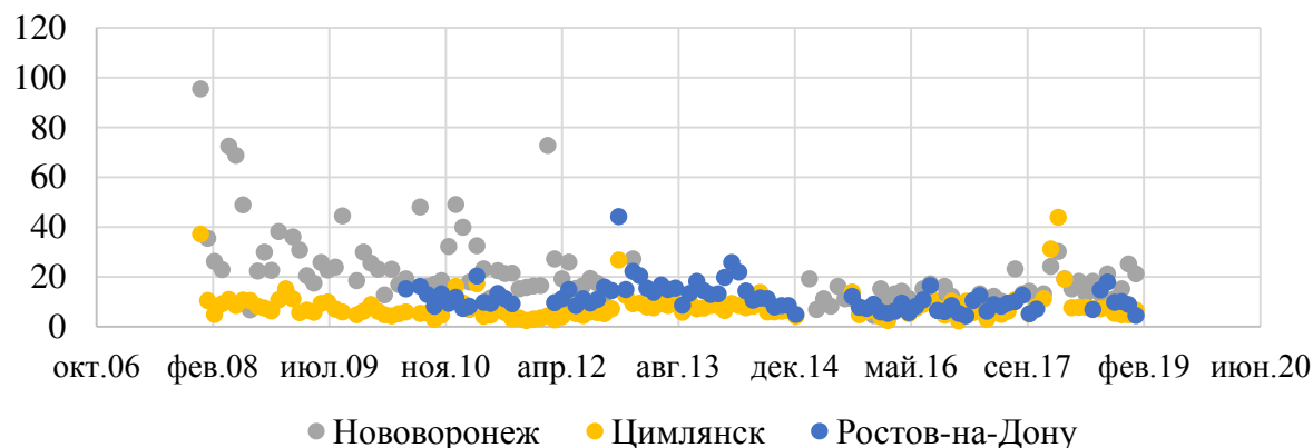
Рисунок 4 – Среднемесячные значения объемной суммарной \beta - активности приземного слоя воздуха, 10^{-5} Бк/м 3 [Monthly mean values of the total volume \beta -activity of the surface air layer, 10^{-5} Bq / m 3 ]
