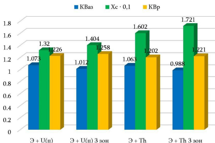
Рисунок 1 – Зависимость KB из K g (коэффициента неравномерности) [Dependence of the coefficient of reproduction on the coefficient of unevenness]
