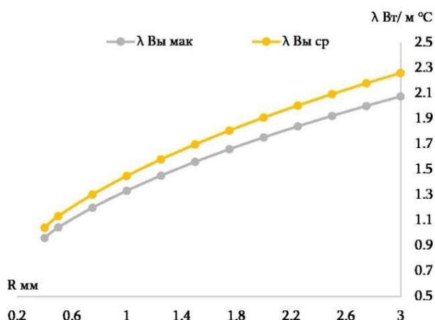
Рисунок 3 – Теплопроводность МОХ-топлива, при выгорании 100 \text{ МВт} \cdot \text{сут/кг} [Thermal conductivity of MOX fuel at a burnout of 100 \text{ MW} \cdot \text{day/kg} ]
