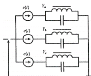
Рис. 1. – Схема для пояснения физики возникновения феррорезонансных явлений [Scheme for explaining the physics of ferroresonance phenomena appearance]
