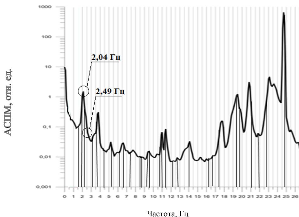
Рис. 5. – АСПМ ВВЭР-440 режим 3 [Autospectral power density of WWER-440 mode 3]
