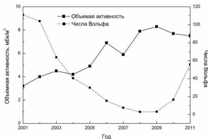
Рисунок 2 – Среднегодовые значения объемной активности 7 Be в приземной атмосфере и чисел Вольфа за период наблюдения с 2001 по 2011 гг. [Average annual values of the volumetric activity of 7 Be in the surface atmosphere and Wolf numbers for the observation period from 2001 to 2011]
