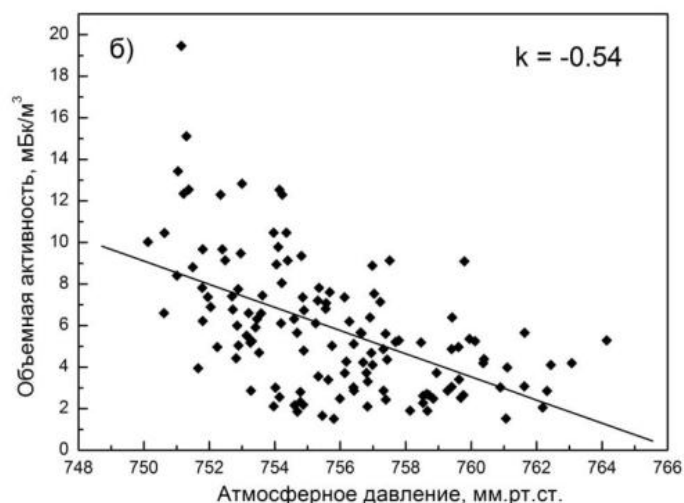
Рисунок 9 – а) Среднемесячные значения объемной активности ^7\text{Be} в приземной атмосфере и атмосферного давления за период наблюдения с 2001 по 2011 гг.; б) Диаграмма рассеяния, иллюстрирующая корреляционную связь среднемесячных значений объемной активности и атмосферного давления за период наблюдений с 2001 по 2011 гг. [a) Monthly mean values of ^7\text{Be} volumetric activity in the surface atmosphere and atmospheric pressure for the observation period from 2001 to 2011; b) Scatter diagram illustrating the correlation between the monthly mean values of volumetric activity and atmospheric pressure for the observation period from 2001 to 2011]
