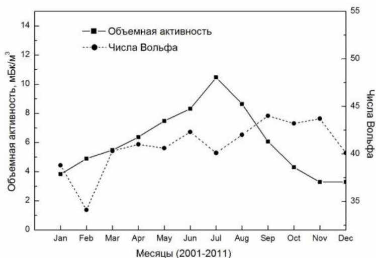
Рисунок 4 – Сезонный ход объемной активности ^7\text{Be} в приземной атмосфере и чисел Вольфа, усредненный за период наблюдений с 2001 по 2011 гг. [Seasonal variation of the volumetric activity of ^7\text{Be} in the surface atmosphere and Wolf numbers averaged over the observation period from 2001 to 2011]
