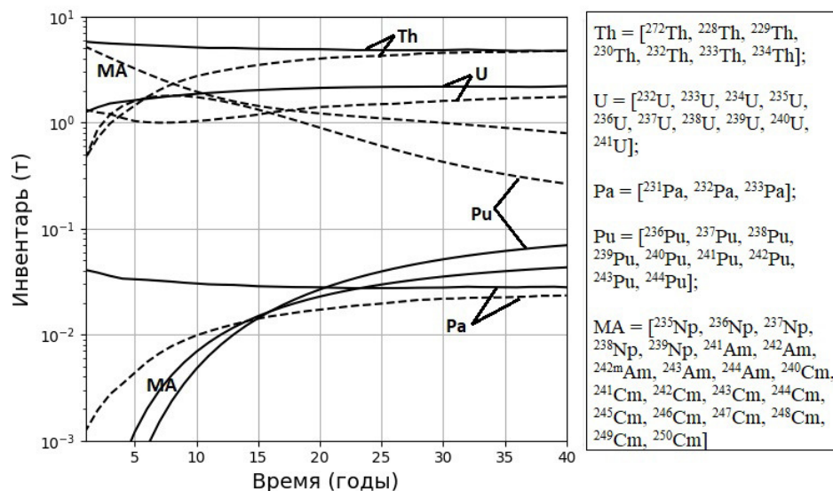
Рисунок 10 – Эволюция важных нуклидов и запасов МА при МА = 0 т (сплошная линия) и МА = 5,82 т (пунктирная линия) для SMSFR при непрерывной переработке (180 сут.) (МА включает Np, Am, Cm) [Evolution of important nuclides and MA stocks at MA = 0 t (solid line) and MA = 5.82 t (dashed line) for SMSFR during online processing (180 days) (MA includes Np, Am, Cm)]
