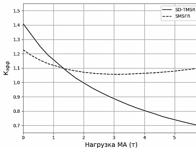
Рисунок 4 – Изменение эффективного коэффициента размножения с нагрузками МА при фиксированной концентрации 233 U для SD-TMSR и SMSFR (статистическая погрешность в K_{эфф} \approx 36 pcm), моделирование без выгорания [Change in effective multiplication factor with MA loads at a fixed concentration of 233 U for SD-TMSR and SMSFR (statistical error in K_{эфф} \approx 36 pcm), simulation without burnout]
