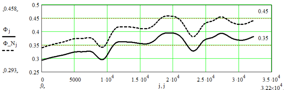
Рисунок 8 – Индикаторы Соколова-Зингера в интервале 61.7 – 62.5 м 3 /ч для нормальных условий эксплуатации ( \Phi_N ) и с внесением 5%-ного возмущения по температуре масла ( \Phi ) [Sokolov-Singer indicators in the range 61.7 – 62.5 cmph for normal operating conditions ( \Phi_N ) and with the introduction of 5% disturbance in oil temperature ( \Phi )]
