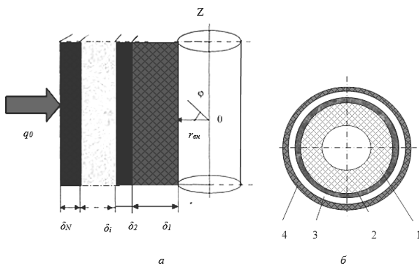
Рисунок 2 – Расчетная схема: a – общая схема для разработки математической модели; b – четырехслойная конструкция; 1 – ТРТ; 2 – капрон; 3 – резина; 4 – материал типа KEVLAR [Design scheme: a – general scheme for developing a mathematical model; b – four-layer construction; 1 – solid propellants; 2 – nylon; 3 – rubber; 4 – Kevlar material]
