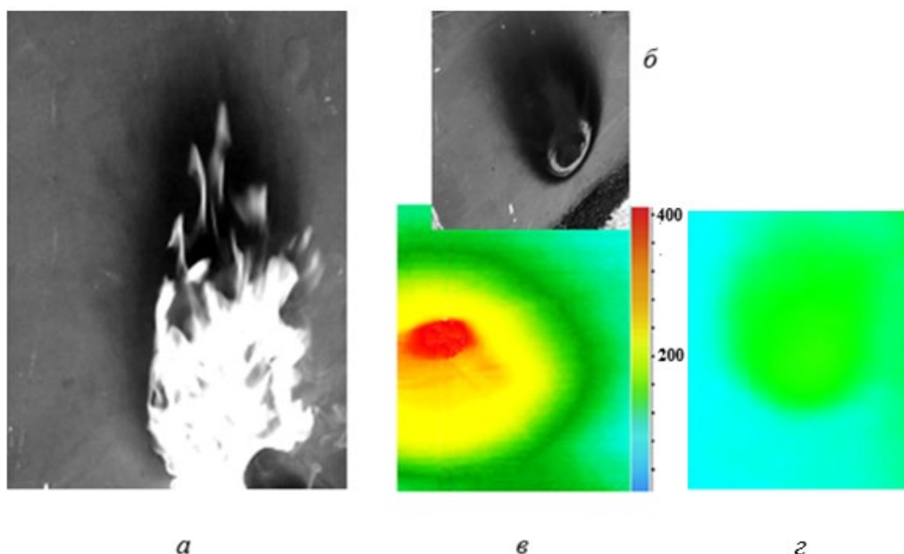
Рисунок 5 – Проведение эксперимента: a – воздействие открытого пламени на образец; б – образец после воздействия; в – изображение внешней поверхности на тепловизоре через 5 секунд после прекращения нагрева; г – внутренняя поверхность на тепловизоре через 5 секунд после прекращения нагрева [Conducting experiments: a – exposure to an open flame on the sample; b – the sample after exposure; c – the image of the external surface on the imager after 5 seconds after stopping heating; d – the internal surface on the imager after 5 seconds after stopping heating]
