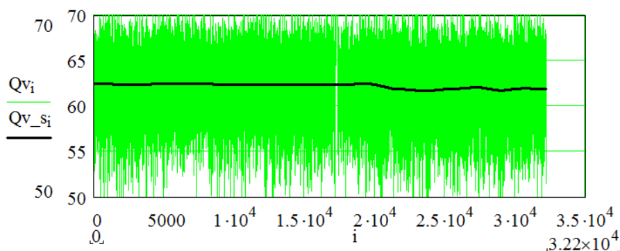
Рисунок 5 – Объёмный расход технической воды при нормальных условиях эксплуатации (м³/ч)
