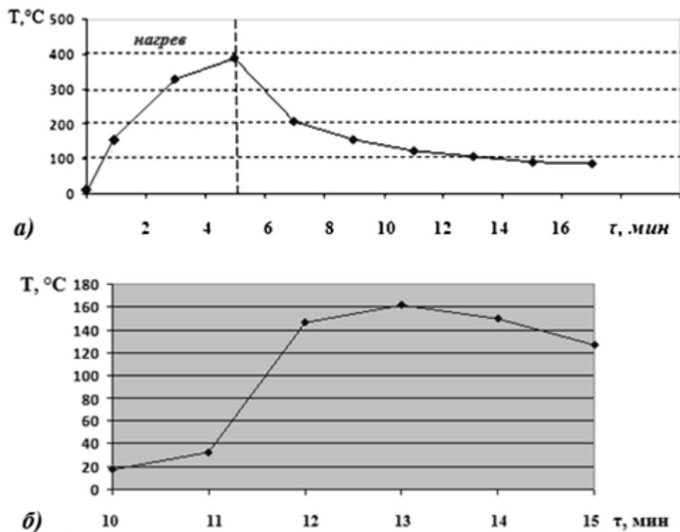
Рисунок 6 – Результаты эксперимента: а – изменение температуры на внешней поверхности образца (время воздействия пламени 330 секунд); б – изменение температуры на внутренней поверхности образца [Experimental result: а – temperature change on the outer surface of the sample (the time of exposure to the flame is 330 seconds), б – temperature Change on the inner surface of the sample]
