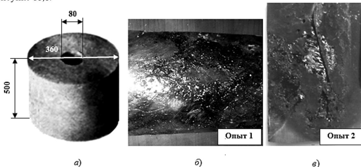
Рисунок 8 – Эксперимент по оценке ядерной взрывобезопасности: а – шашка твердого топлива; б, в – фрагменты конструкции модели после проведения эксперимента [An experiment on the estimation of nuclear explosion: a – solid fuel stick; b, c – fragments of the model structure after the experiment]
